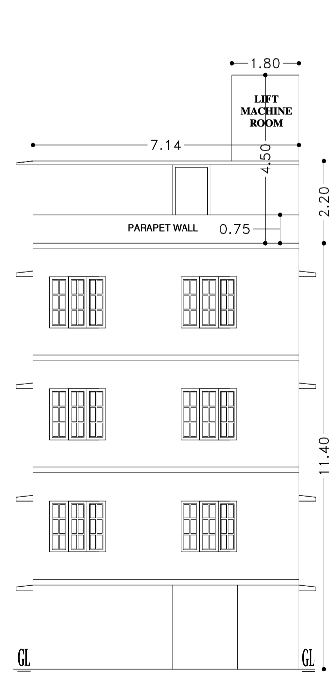
ELEVATION
